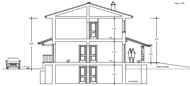
SEZIONE A-A
