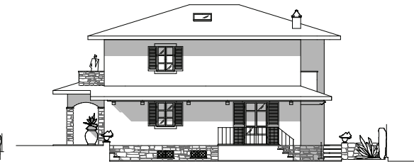
PROSPETTO OVEST
