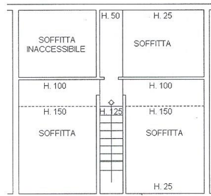
PIANO SECONDO
