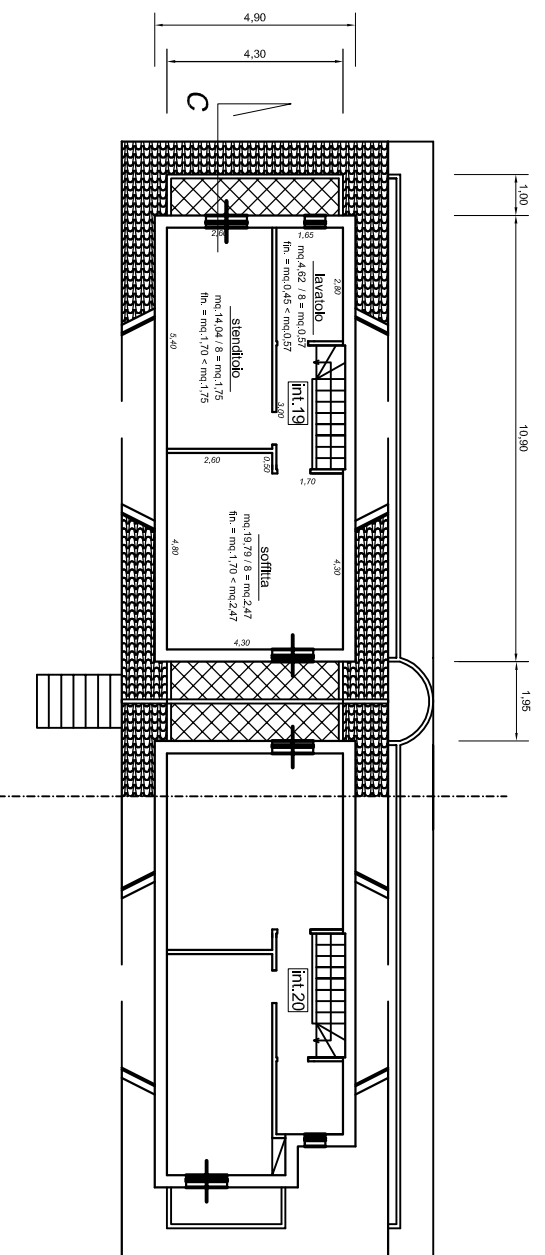
PLANIMETRIA PIANO SOTTOTETTO - corpo "C" - rapp. 1:100
