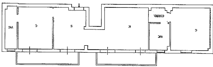
Piano primo h. 3,10 mt
