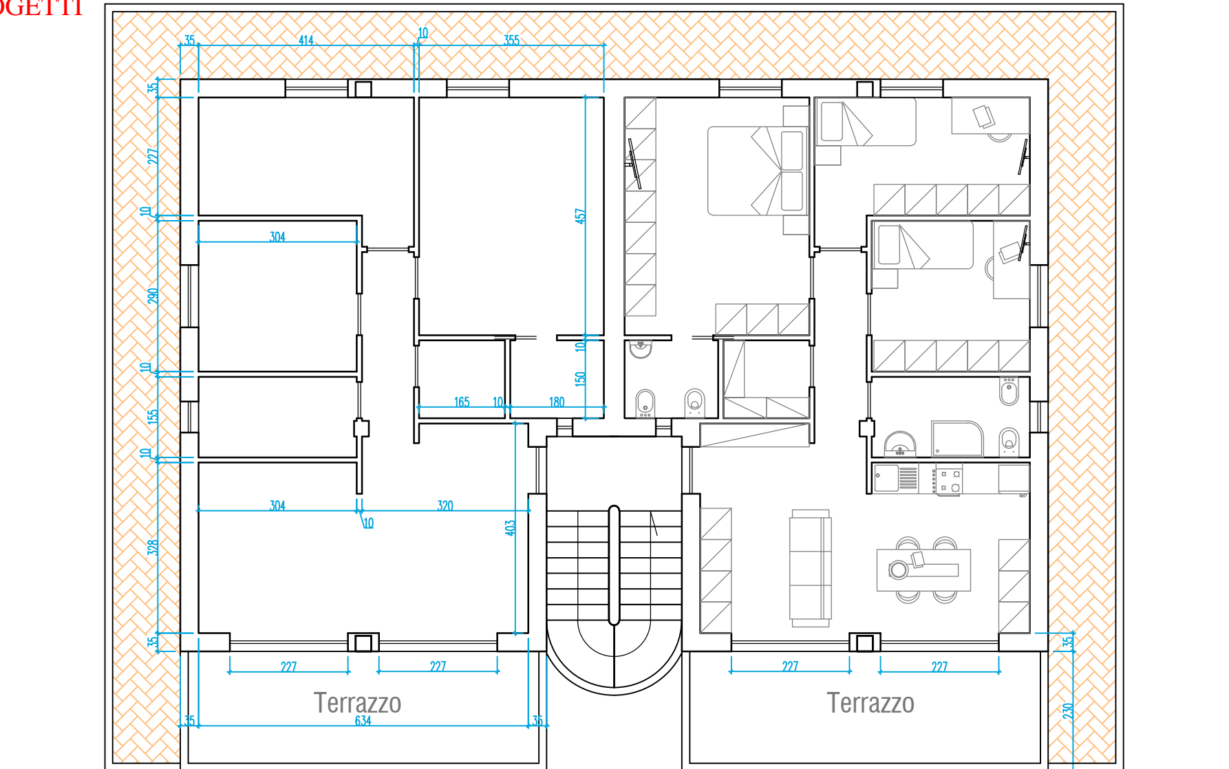
PLANIMETRIA TIPO quadrilocale mq 86.00 + balcone
