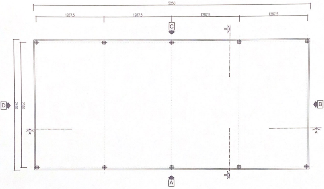
PIANTA PIASTRINI
