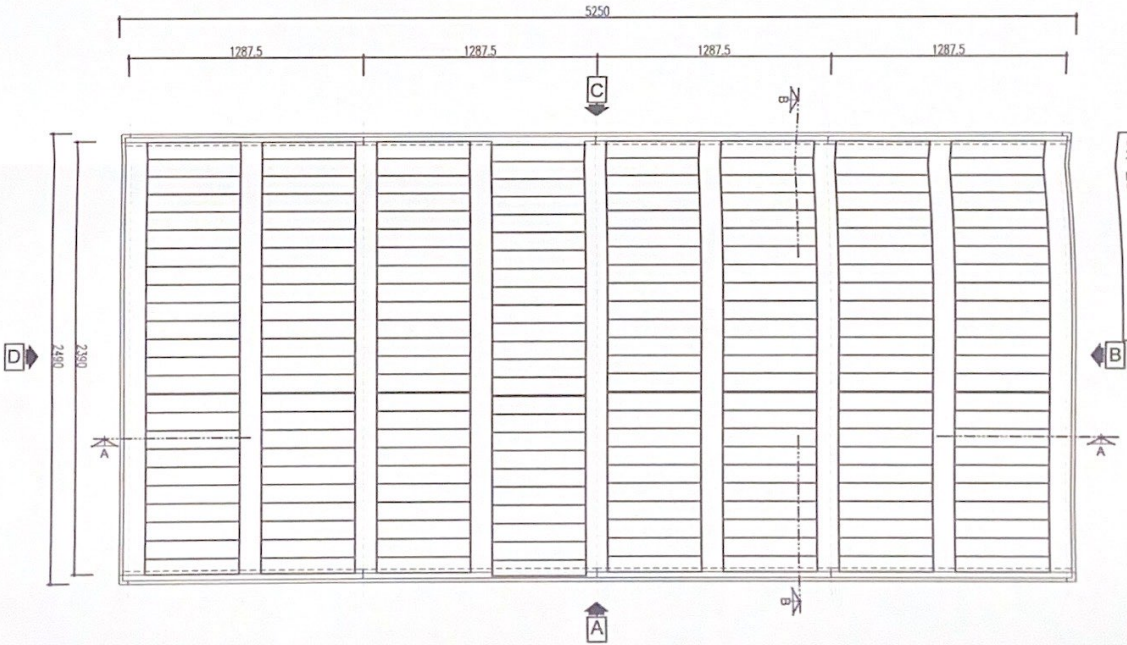
PIANTA COPERTURA sv. 20+30+50 kg/mq.
