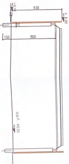
SEZIONE B-B
