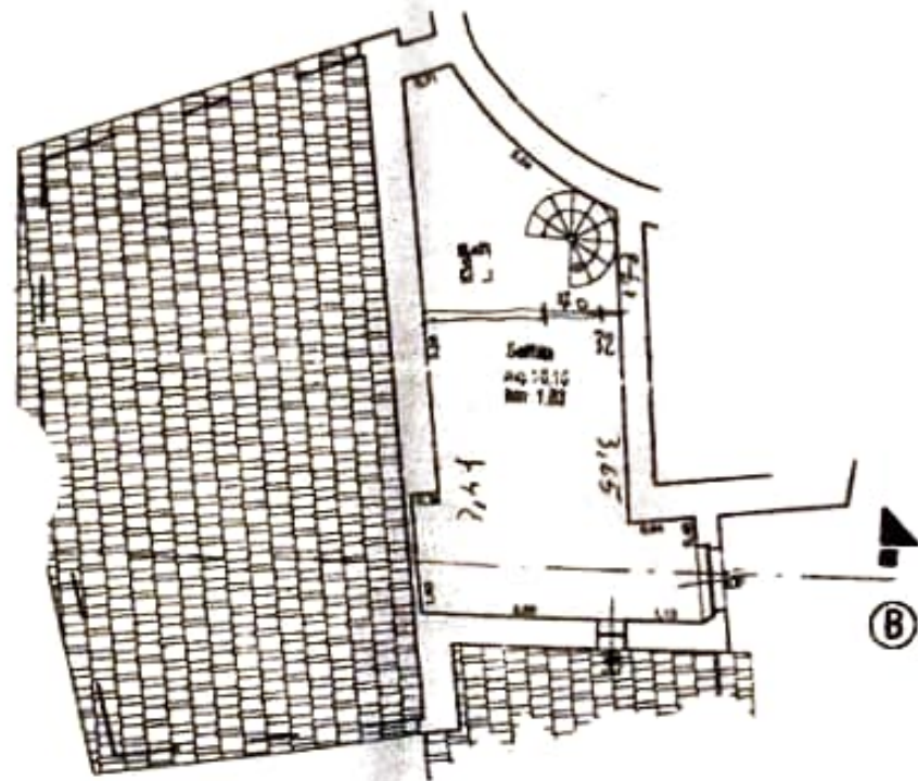
PIANO SOFFITTA STATO VARIATO
