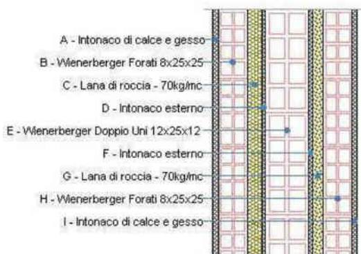
M4 - Parete divisoria tra alloggi (sp. 40 cm)
