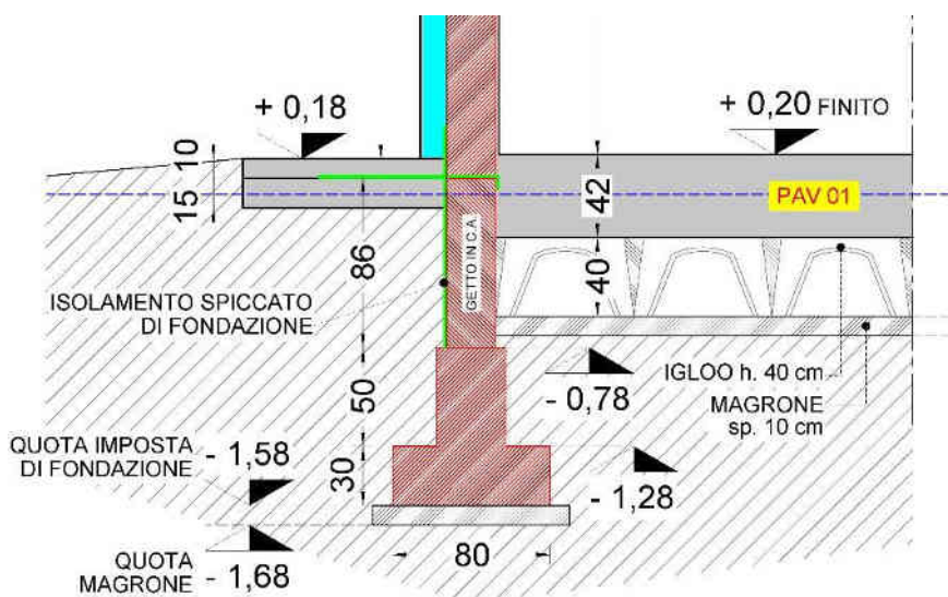
PARTICOLARE COSTRUTTIVO TIPO
